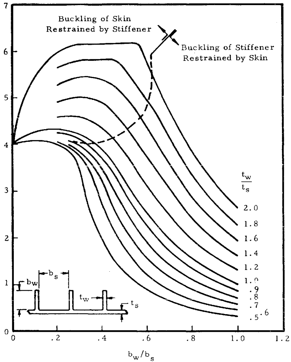
(a) Web Stiffeners 0.5 < t_w/t_s < 2.0
